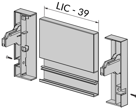
Montage de la façade Front profile assembly
