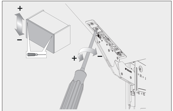
Réglage de la porte haut et bas Door adjustments up and down
