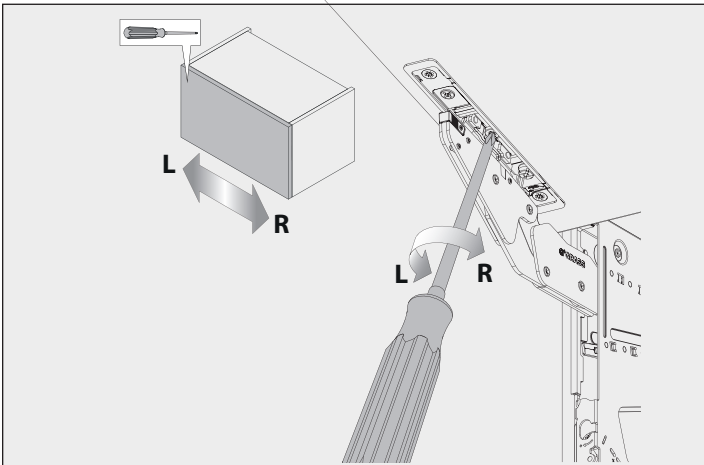
Réglage de la porte gauche droite Right and left door adjustment
