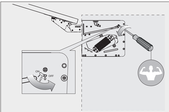
Désactiver la fermeture amortie Door angle adjustment
