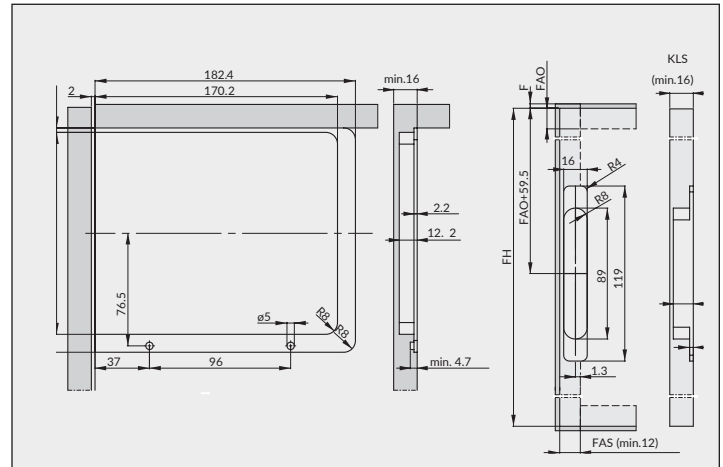
Machinage pour montage encastré Side and door machining for inset mounting
