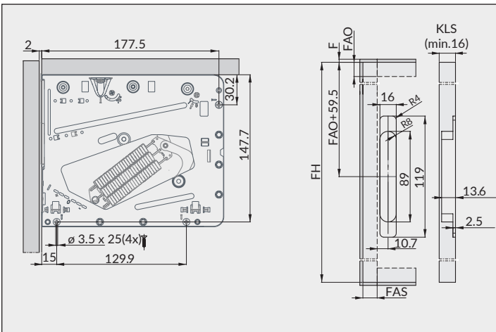
Montage en surface et machinage de la porte Applied mounting and door machining
