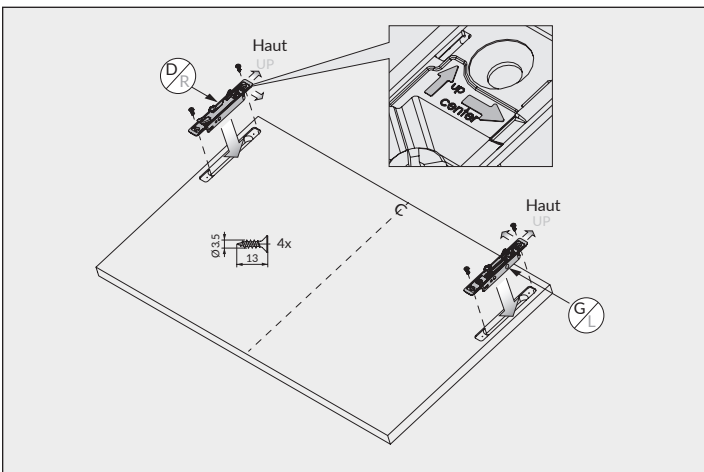
Montage des plaques dans la porte Mounting plates in the door
