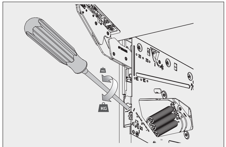
Régler la tension de la porte Door tension adjustment
