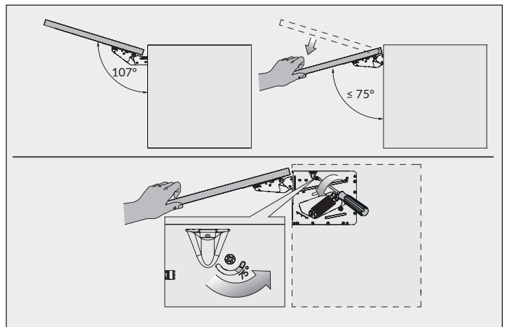
Ajustement de l'angle de l'ouverture Door angle adjustment
