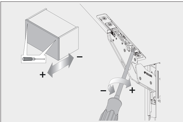
Réglage de la porte avant arrière Door depth adjustment
