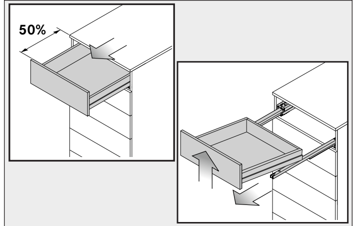
Ouvrir le tiroir à mi-course et soulever l'avant pour l'enlever. Open the drawer halfway, lift off the drawer to remove.
