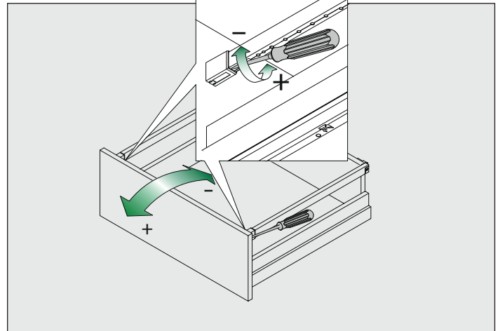
Inclinaison de façade sur tiroir H90 avec tubes Front tilt on a H90 drawer with lateral tubing
