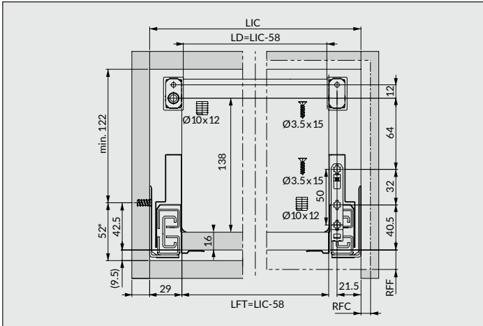
Montage type du tube sur tiroir H90 Tube installation on a H90
