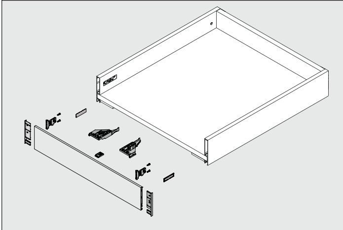
Fixer les attaches et les embouts sur la façade d'aluminium. Fix the front brackets and endcap on the aluminum drawer front.
