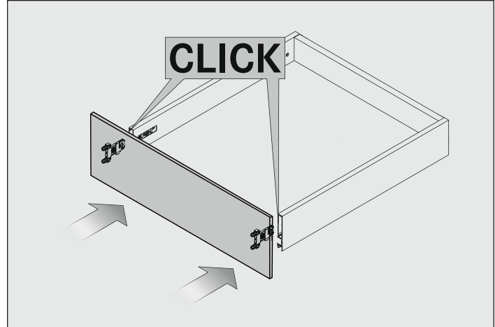
Monter la façade sur le tiroir Mount the front on the drawer
