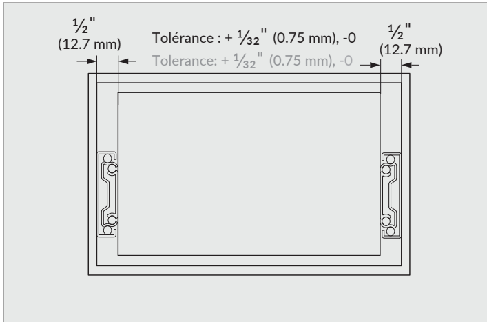
Espacement requis pour la coulisse de chaque côté du tiroir Minimum displacement required on each side of the drawer
