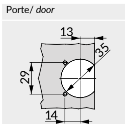
Schémas de perçage Drilling pattern
