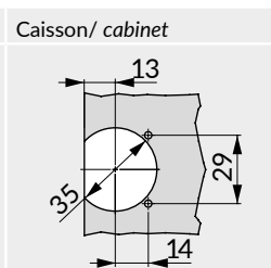
Profondeur de perçage Drilling depth
