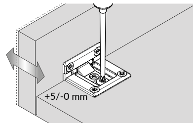
Réglage de la profondeur Depth adjustments
