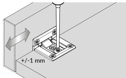
Réglage latéral Lateral adjustments
