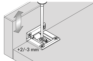
Réglage en hauteur Height adjustments
